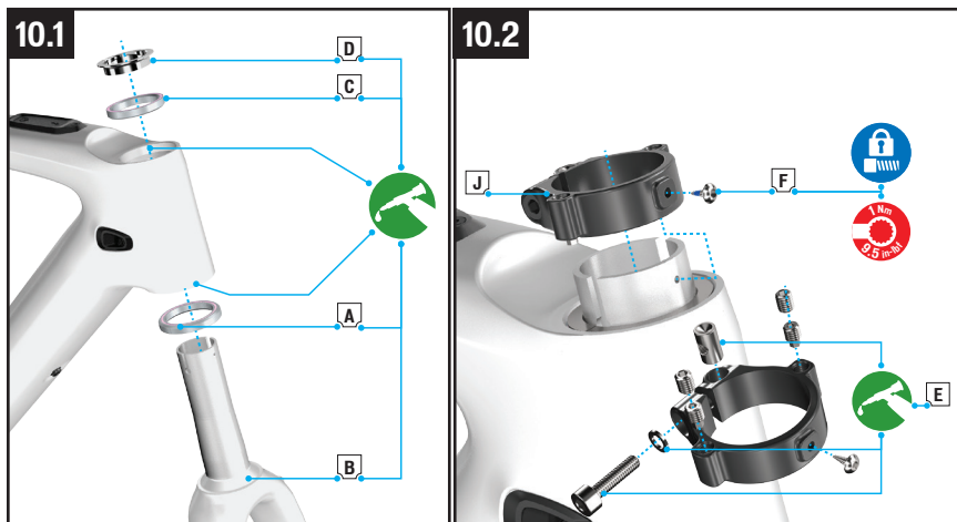
Obr. 10.1: Naneste vazelínu a potom namontujte spodné ložisko (A) na vidlicu (B). Vložte vidlicu do hlavovej trubky, potom namažte a namontujte horné ložisko (C) a kompresný krúžok (D) na stĺpik vidlice.
