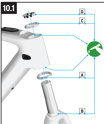
Abb.10.1: Schmieren Sie das untere Lager (A) und bringen Sie es an der Gabel (B) an. Setzen Sie die Gabel in das Steuerrohr ein, fetten Sie das obere Lager (C) und den Kompressionsring (D) und montieren Sie beide am Steuerrohr.
