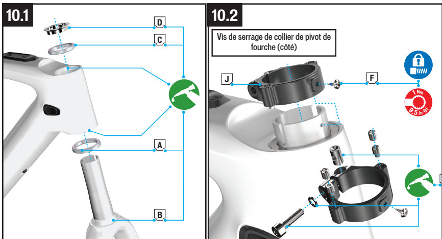
Fig.10.1 : Graissez puis installez le roulement inférieur (A) sur la fourche (B). Insérez la fourche dans la douille de direction puis graissez et installez le roulement supérieur (C) et la bague de compression (D) sur le pivot de fourche.
